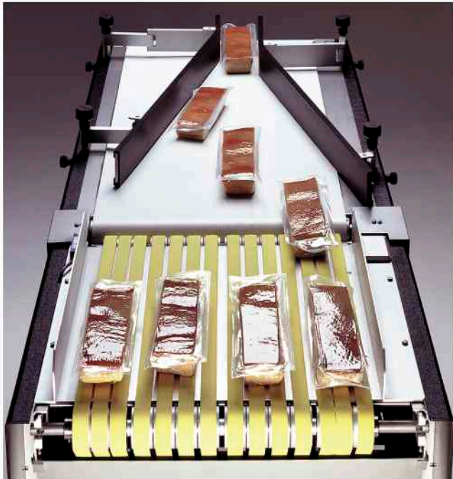
De flexibele sturing van de transportbanden brengt tot 6 lijnen op lijn
