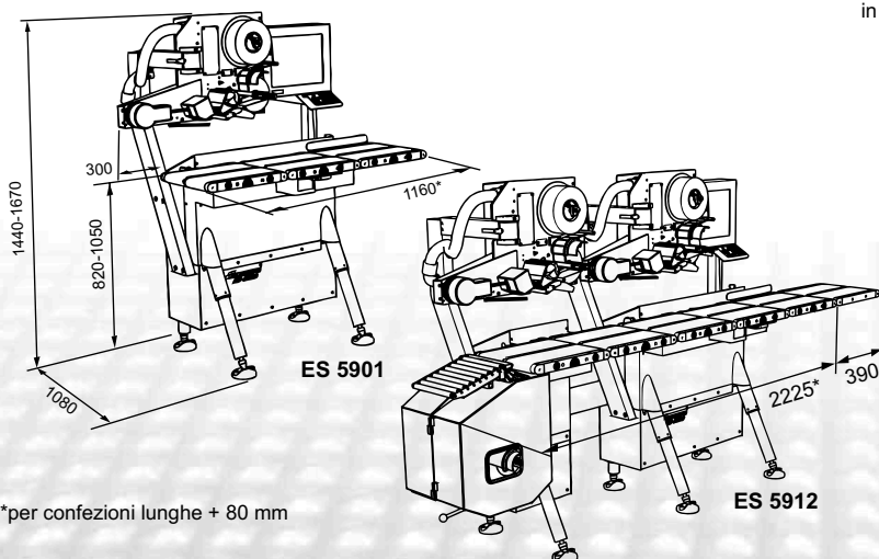
Nastro di carico / unità separazione pacchi opzionale
