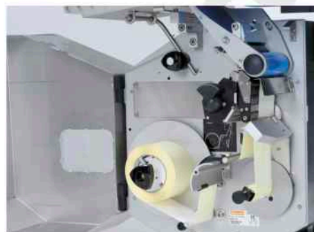
Stampante inferiore con bobina fino a 210 mm in cassa protetta dagli spruzzi d'acqua
